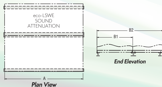
eco-LSWE Attenuation
